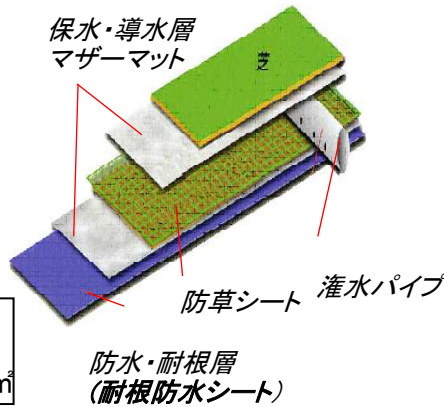
花壇構造図
