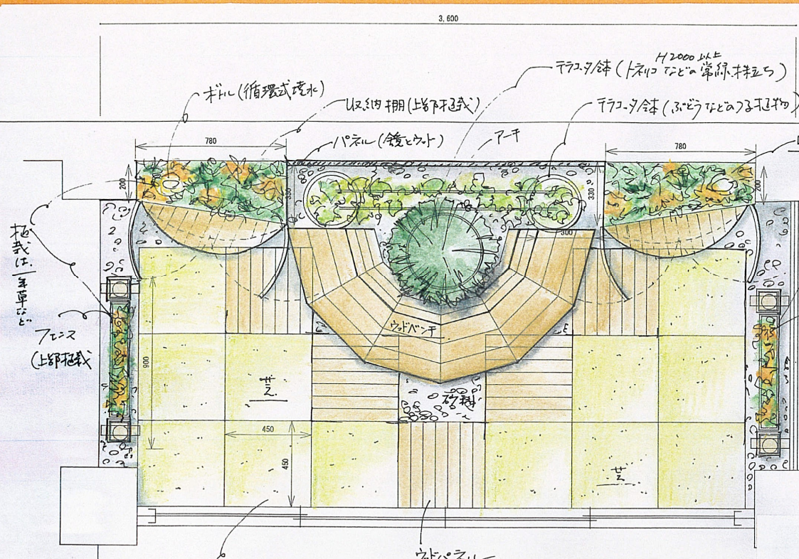
平面図 1/20 2003.7
