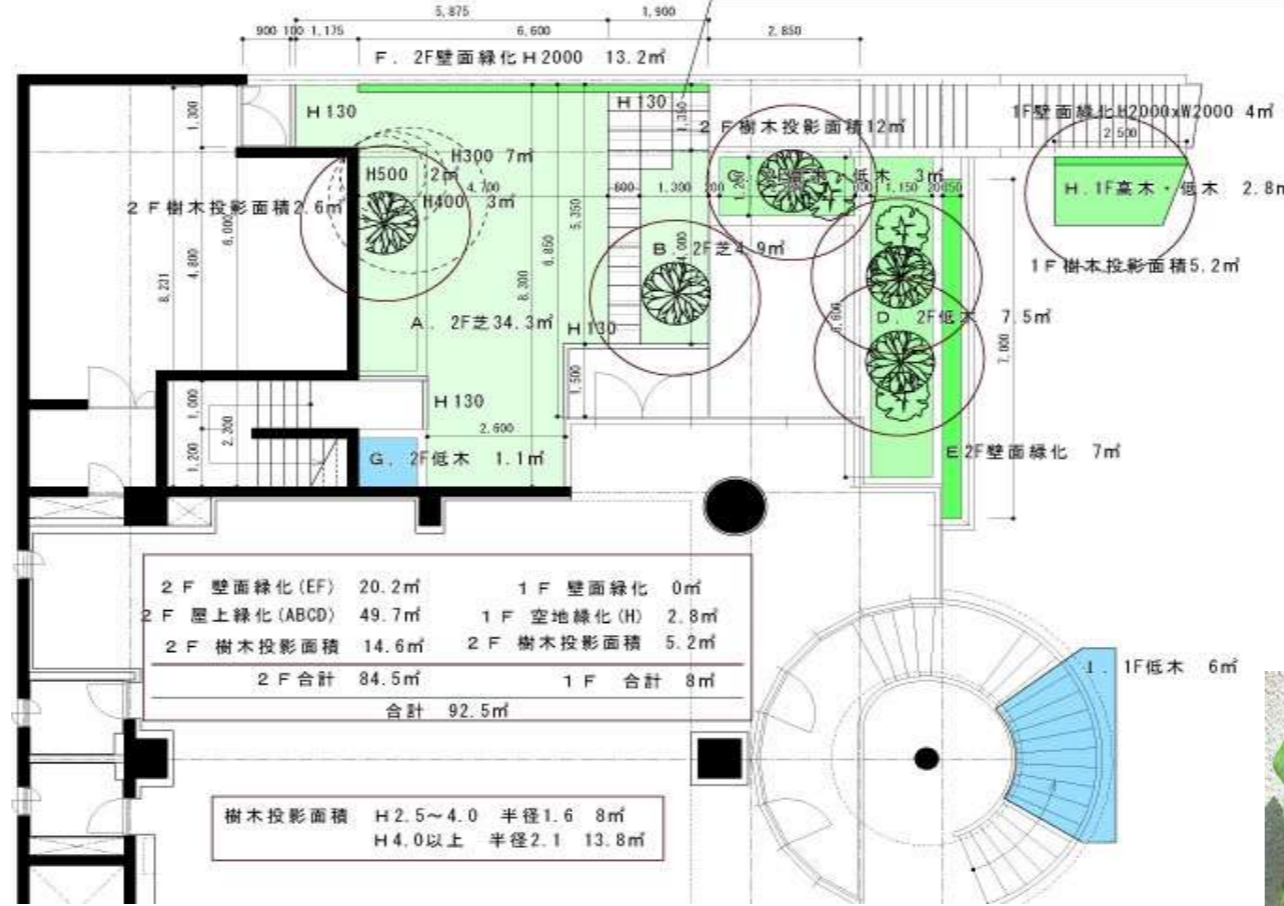
2016-12-11casas様プラン1平面図 1/100 2016-11-11
