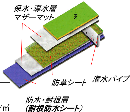
花壇構造図
