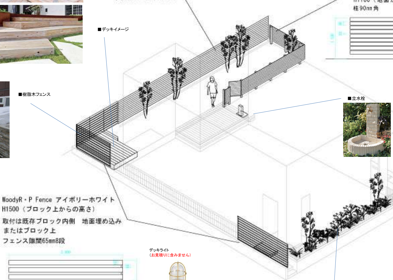
木横板フェンスH1500
